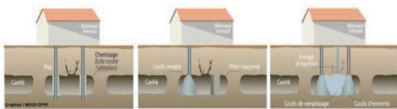
Fig. 38 : Protection active contre les cavités souterraines. ( www.Prim.net )
